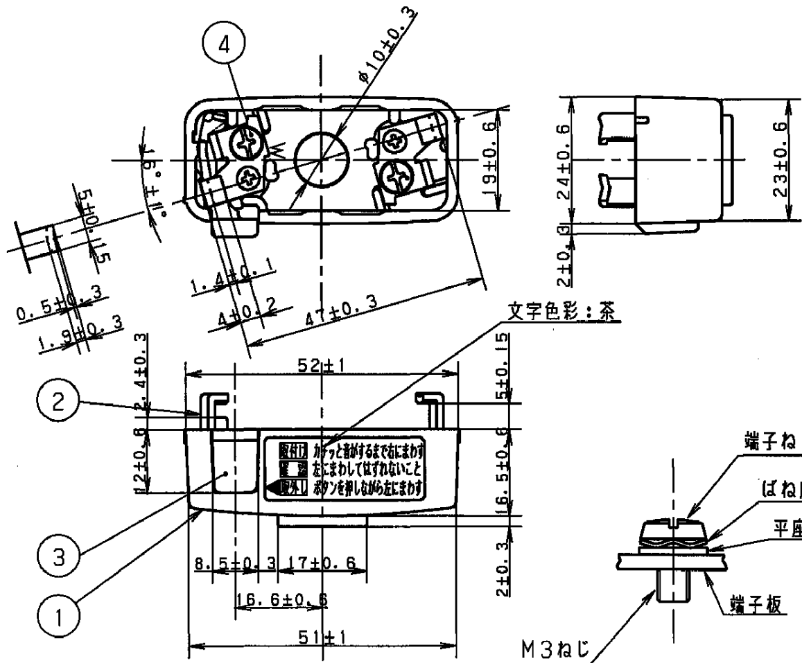
端子部詳細図 (2:1)
