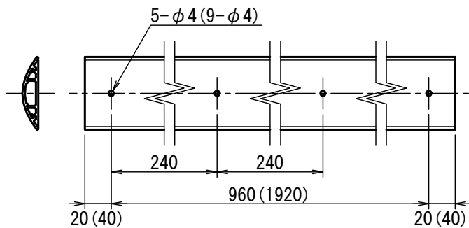
製品裏面釘穴図
