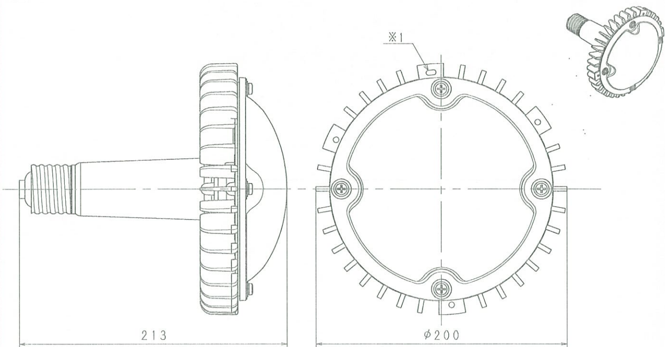
※1 落下防止ワイヤ用取付穴
