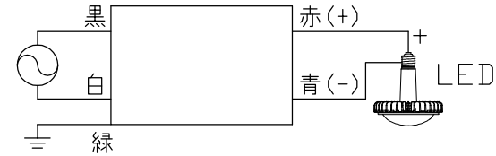
取付条件
