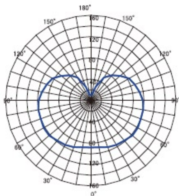
配光曲線図
