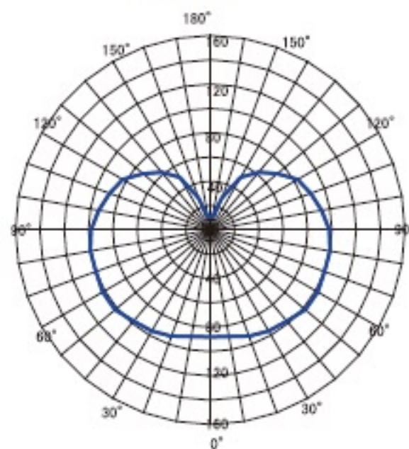
配光曲線図
