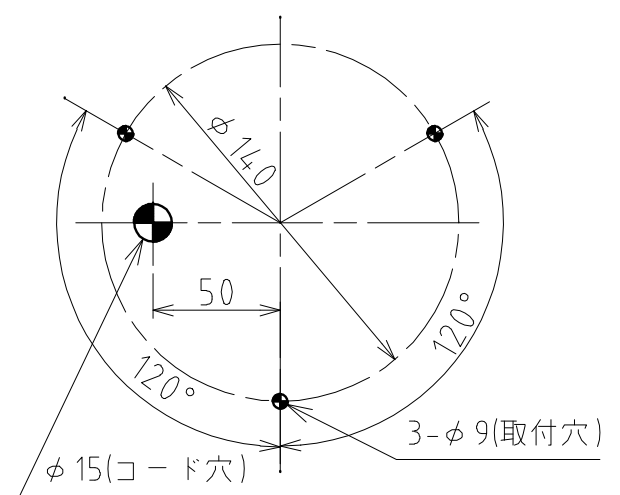
正面方向 取付寸法図（取付表面側より加工の場合）
