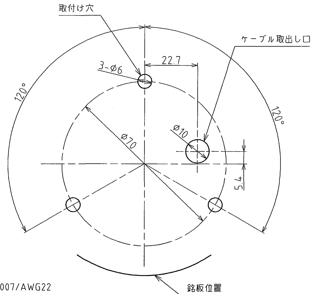
取付面寸法図
