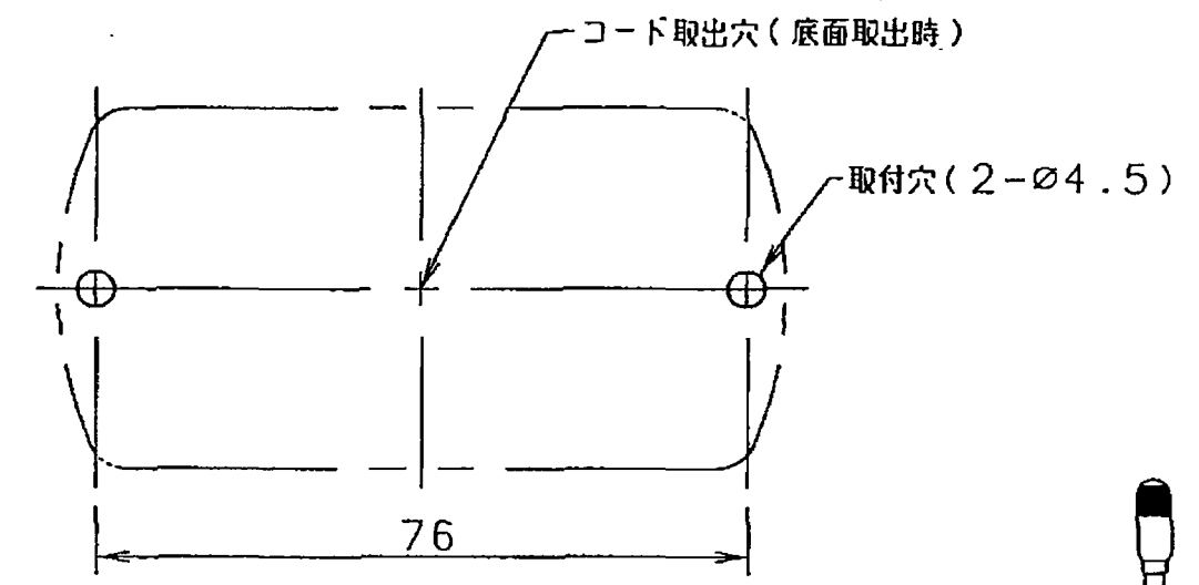
取付面寸法図
