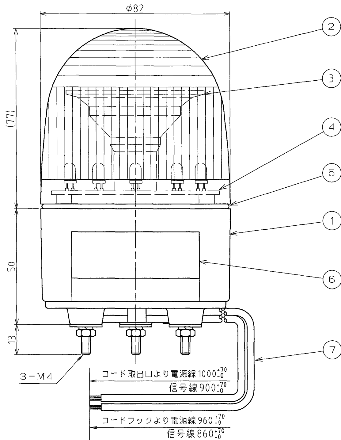
外観寸法図
