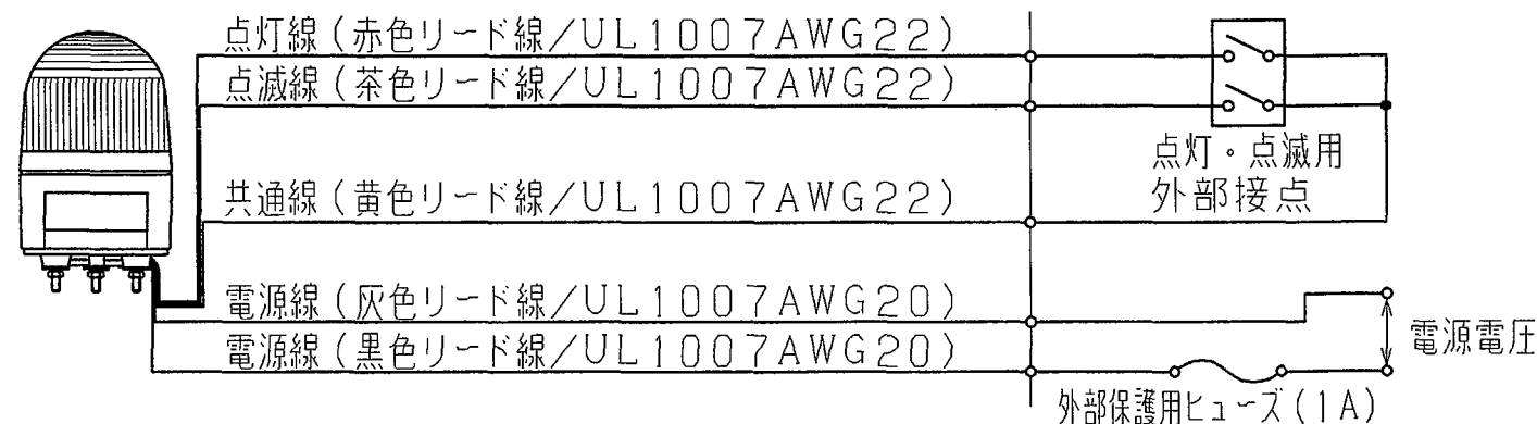
配線図
