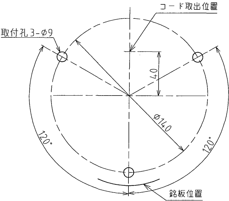
取付面寸法図 (尺度 1:2)
