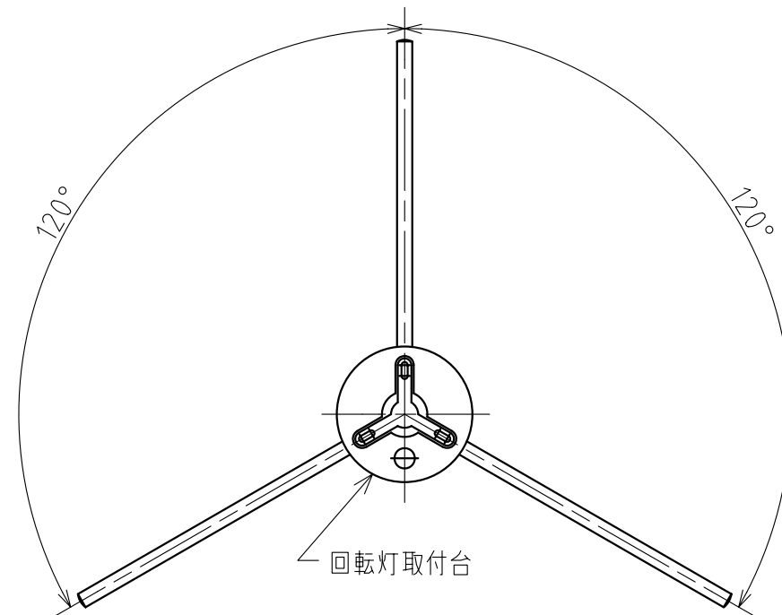
上視図
