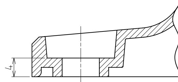
A-A'部断面図 (2:1) Cross section A-A'(2:1)
