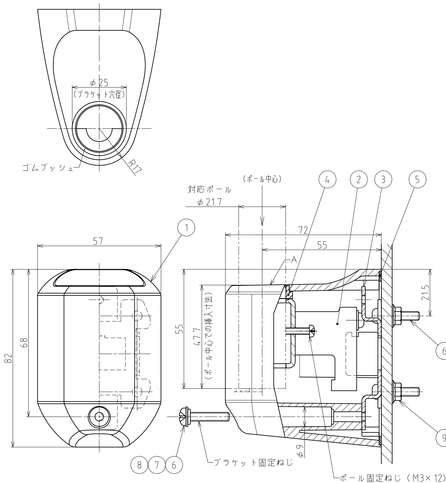
外観寸法図
