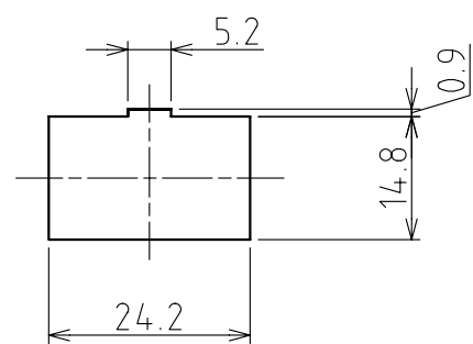
取付金具コード穴寸法 (コネクタ取付穴)
