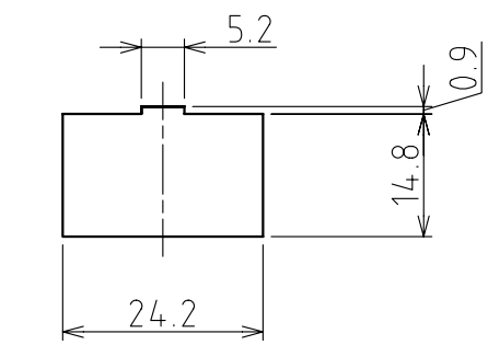
取付金具コード穴寸法 (コネクタ取付穴)
