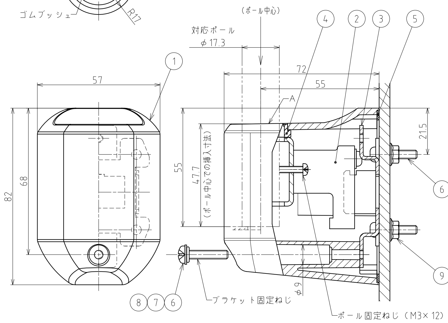
外観寸法図
