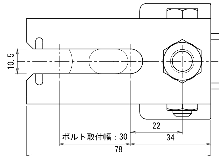
底面図
