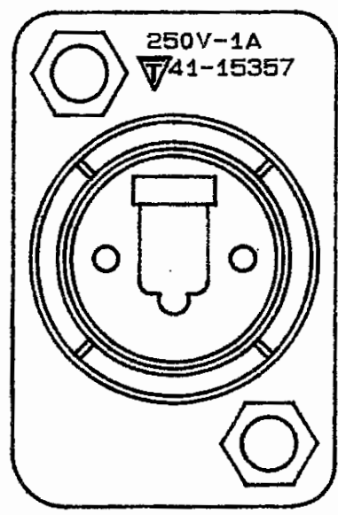
A 詳細図
