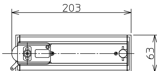
取付部
