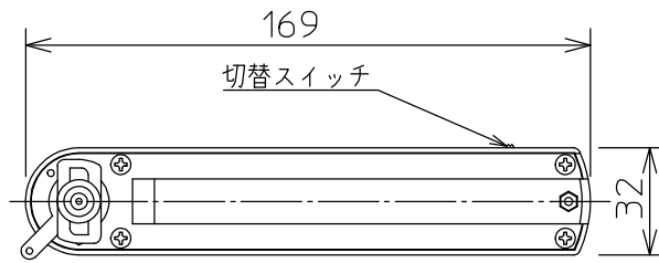
取付部
