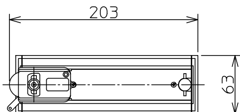
取付部
