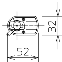
取付部
