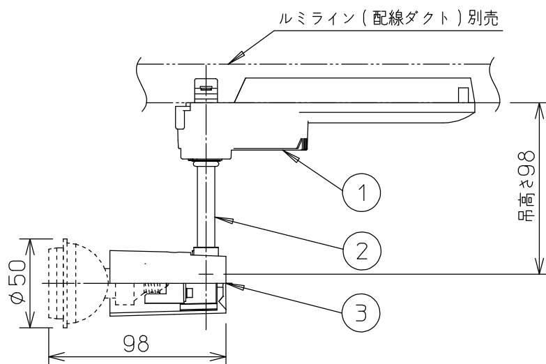
取付部
