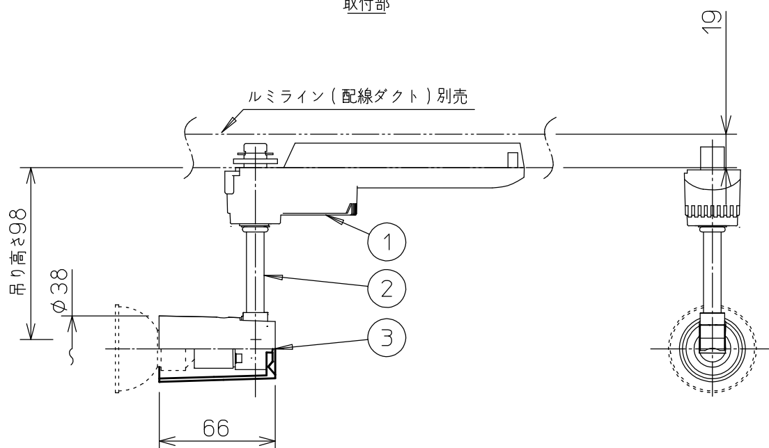
取付部
