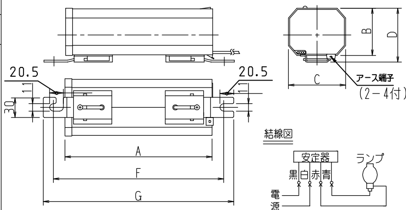
寸法表
