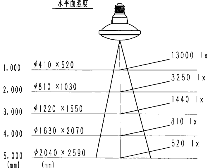
水平面照度
