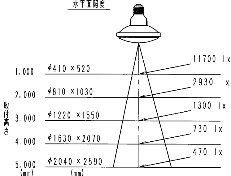
水平面照度
