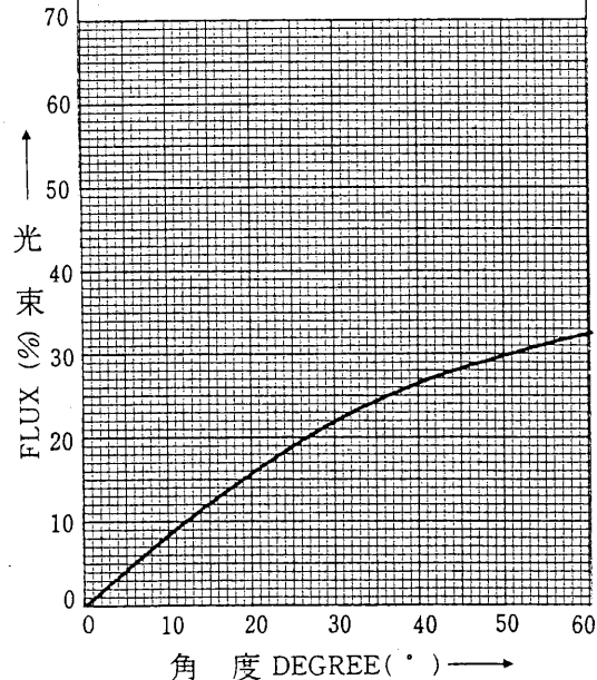
光束累積曲線 ACCUMULATIVE FLUX CURVE
