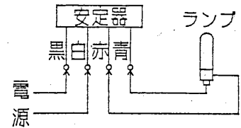
結線図
