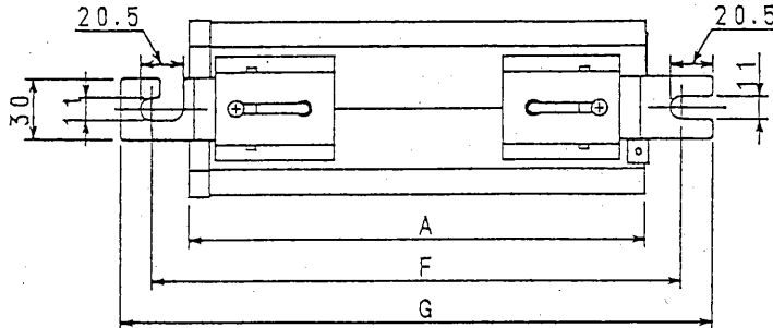
寸法表
