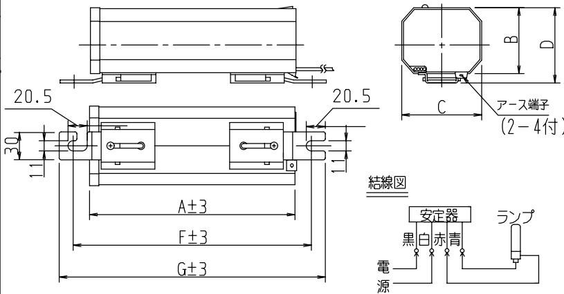
寸法表
