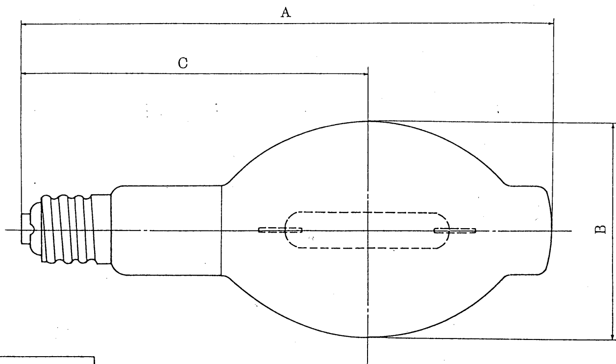
性能表
