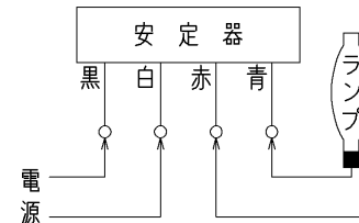
結線図
