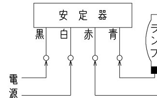
結線図
