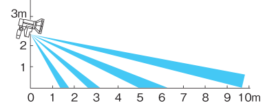
側面図(2.5m取付時)
