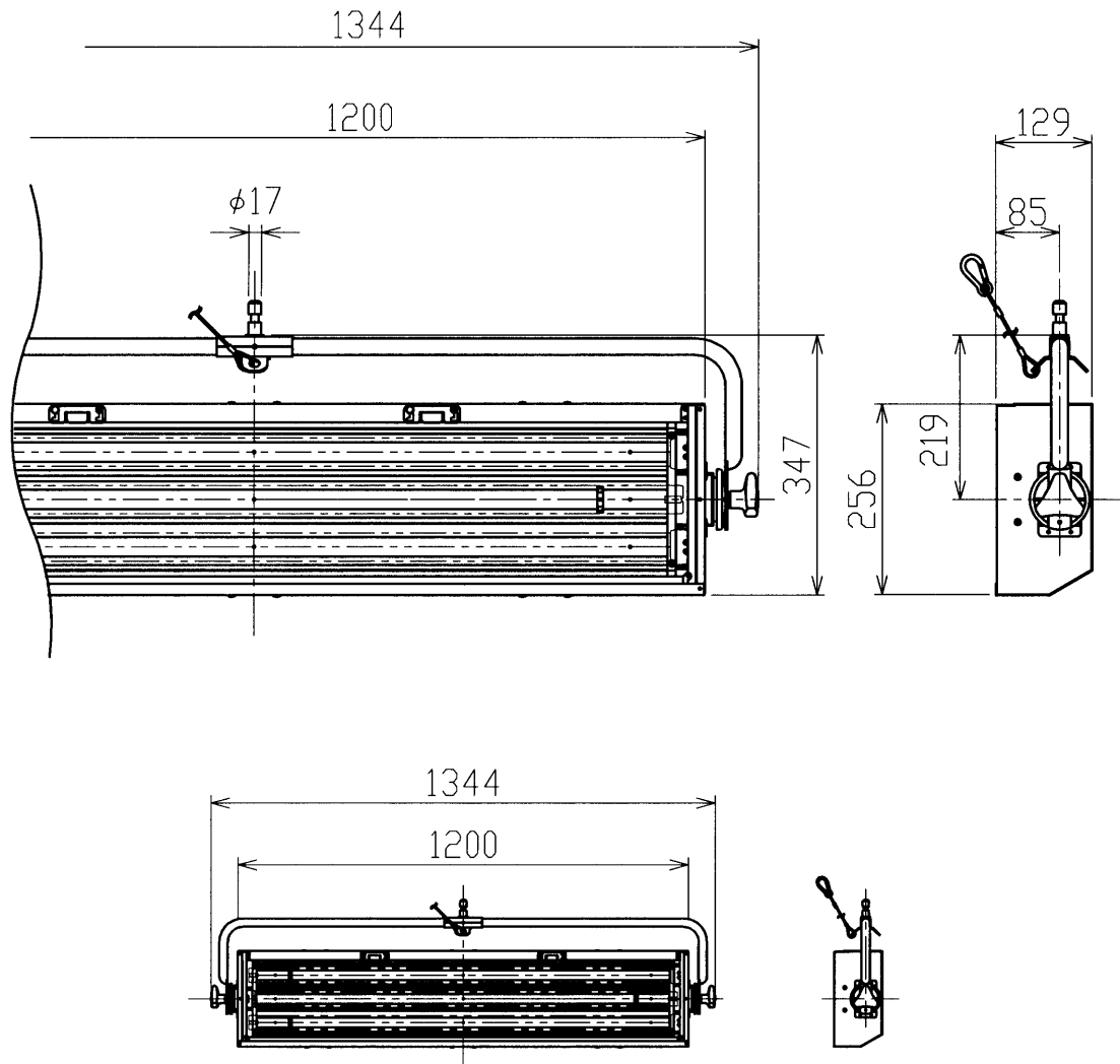
全体図 S=1/20
