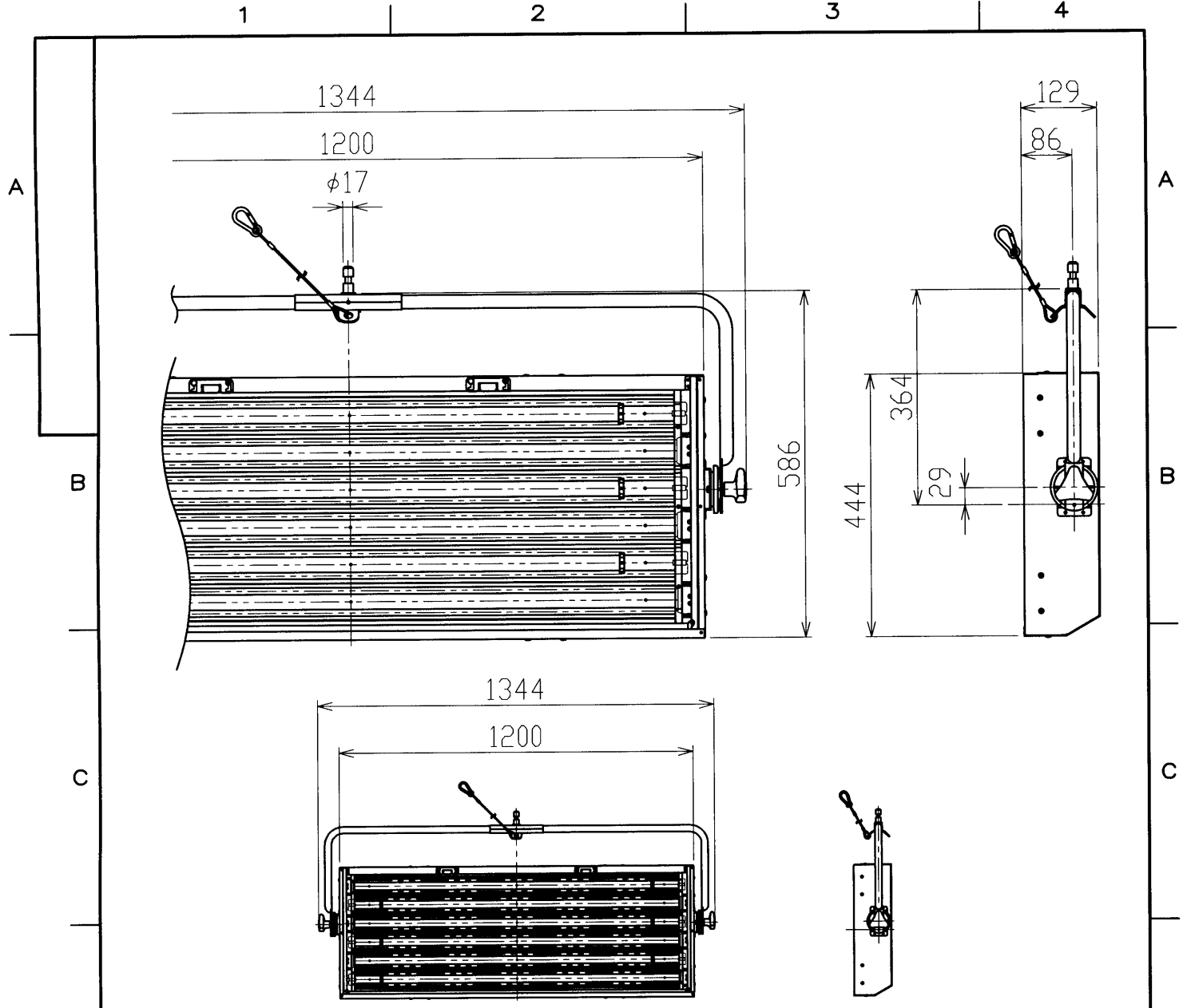
全体図 S=1/20
