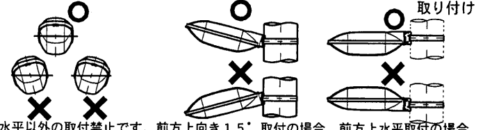
水平以外の取付禁止です。前方上向き15°取付の場合 前方上水平取付の場合
