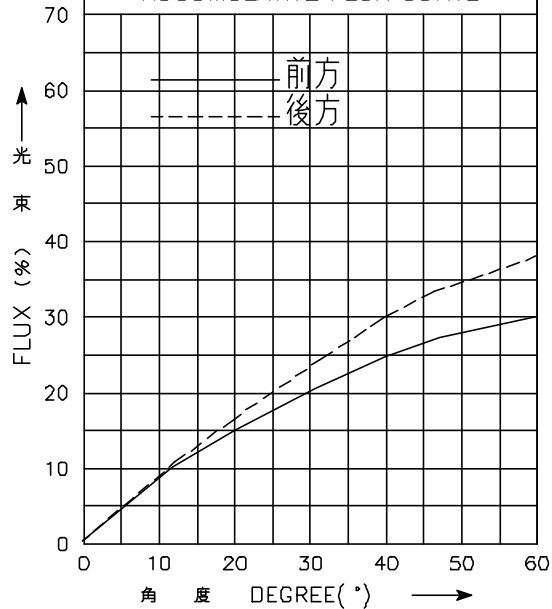
光束累積曲線 ACCUMULATIVE FLUX CURVE
